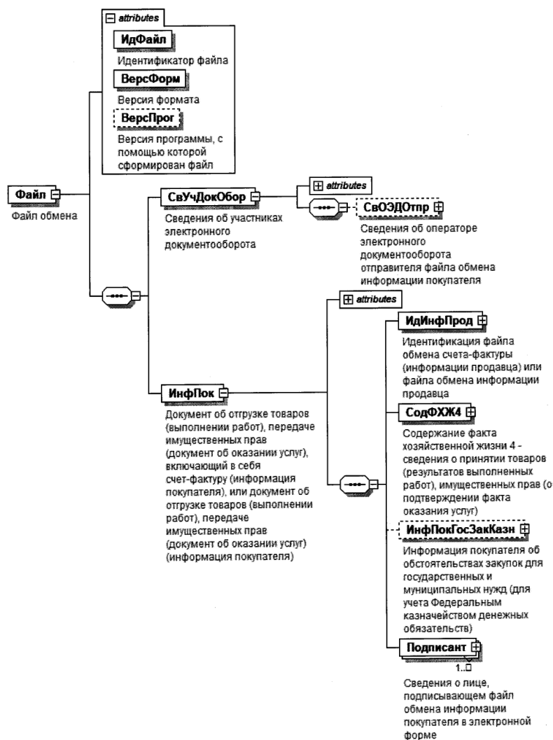
Рисунок 2. Диаграмма структуры файла обмена
