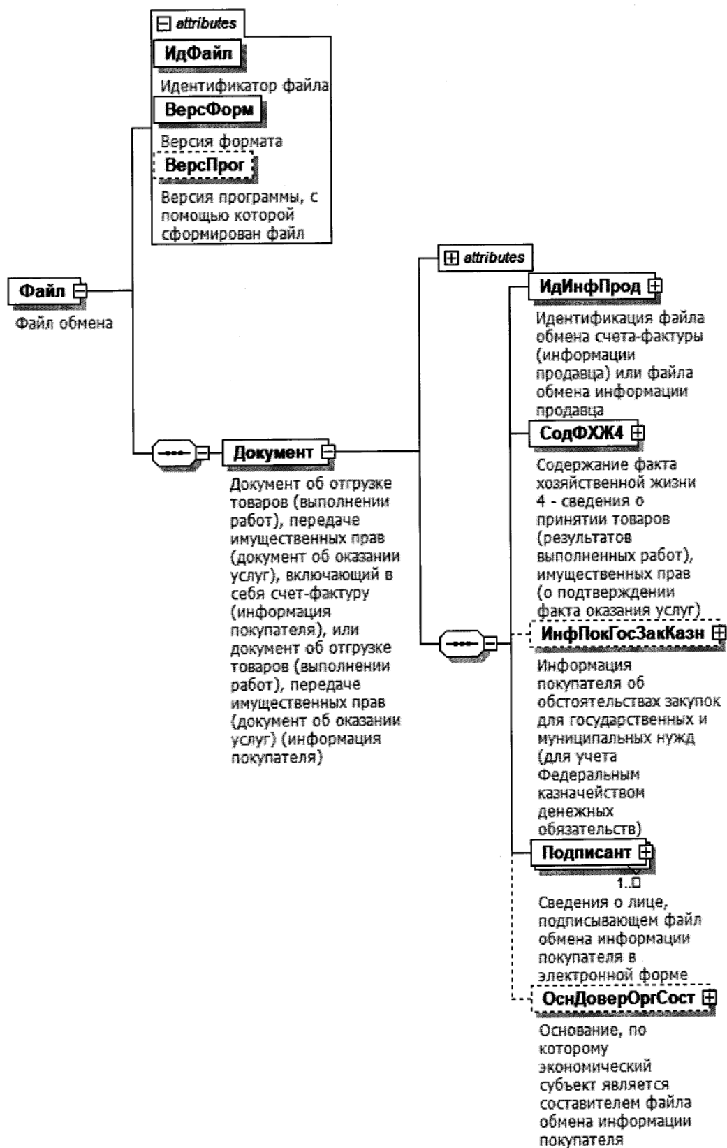
Рисунок 2. Диаграмма структуры файла обмена
